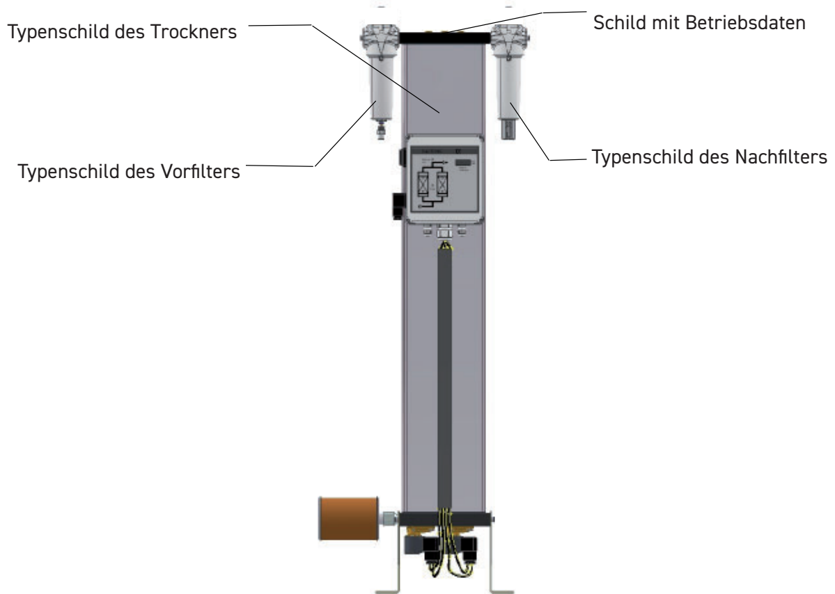
Vorderansicht
